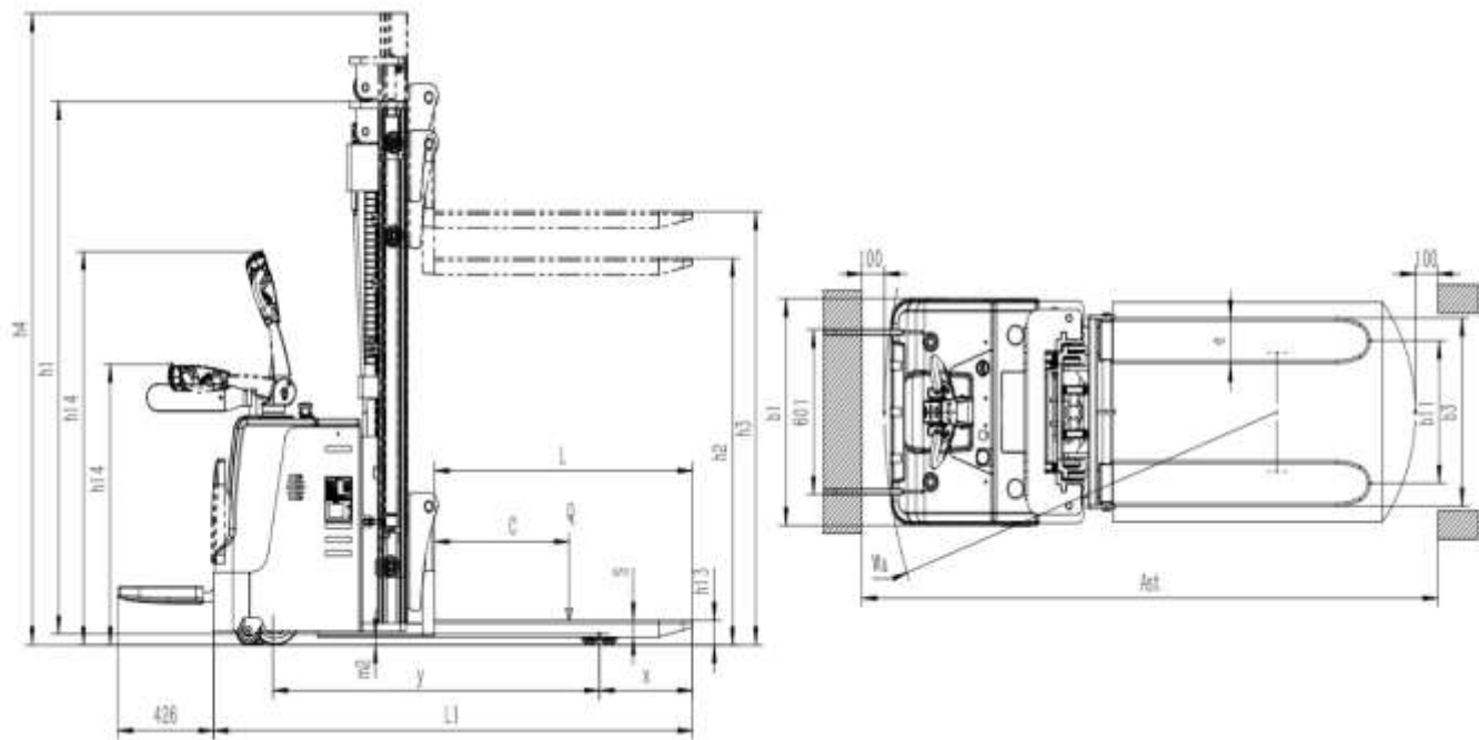
Рис. 1 - Габаритные размеры
