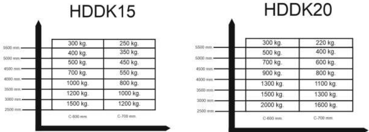
Рис. 2 – Кривые грузоподъемности
